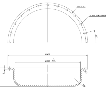
Pieza embutida en chapa de ocho para válvulas industriales
